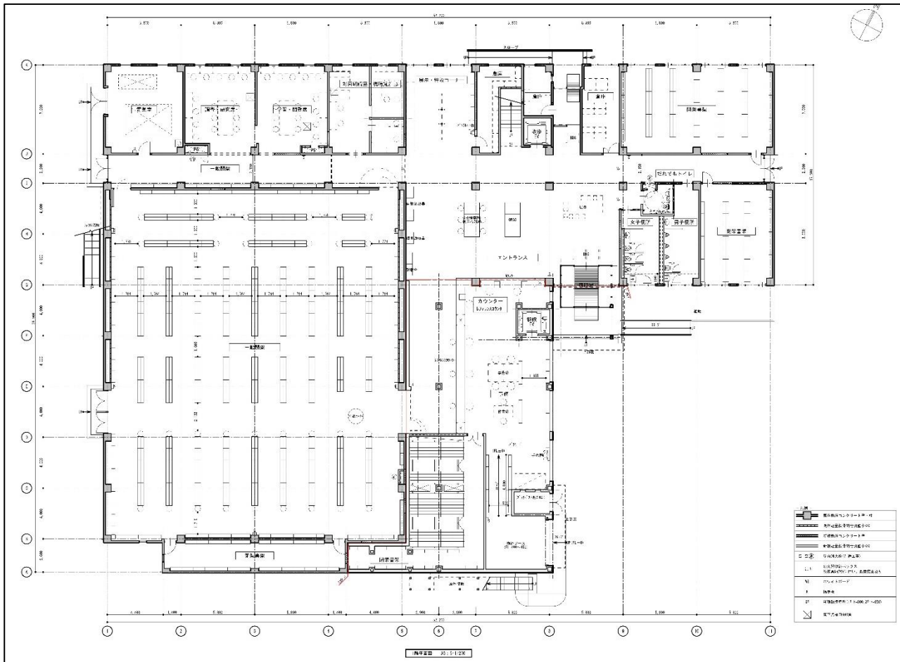
■ 平面図 1階
